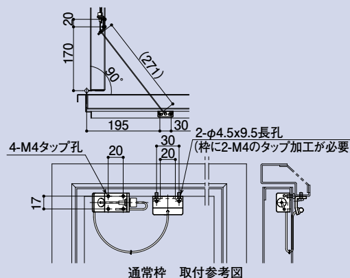
通常枠 取付参考図
