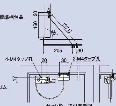
サッシ枠 取付参考図
