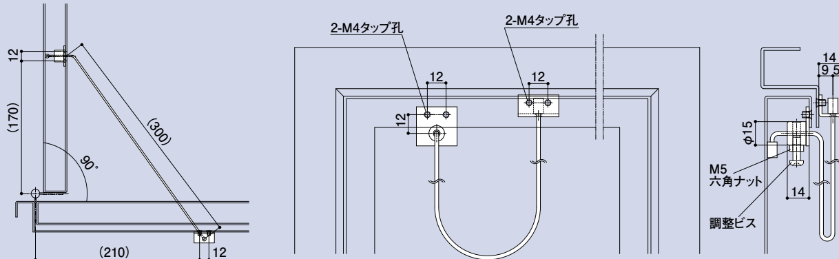
取付参考図
