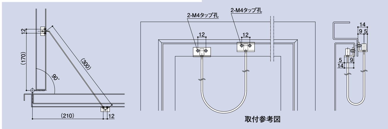
ワイヤーストッパー
