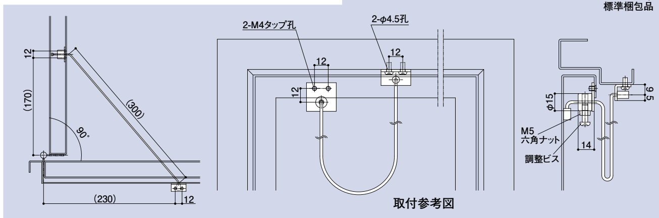
ワイヤーストッパー(長さ可変仕様)
